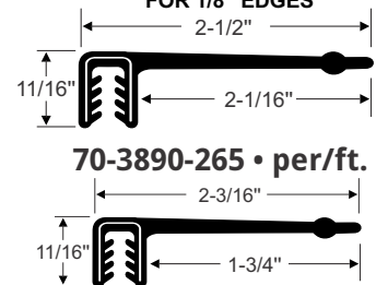
70-3889-265 • per/ft.
