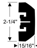
EXTRUSION 70-4093-247 • per/ft.
