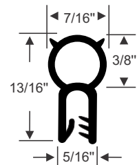
70-3854-245 • per/ft.
